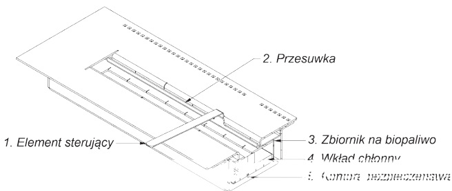
Rys. 1. Biopojemnik Spark700 - przekrój
